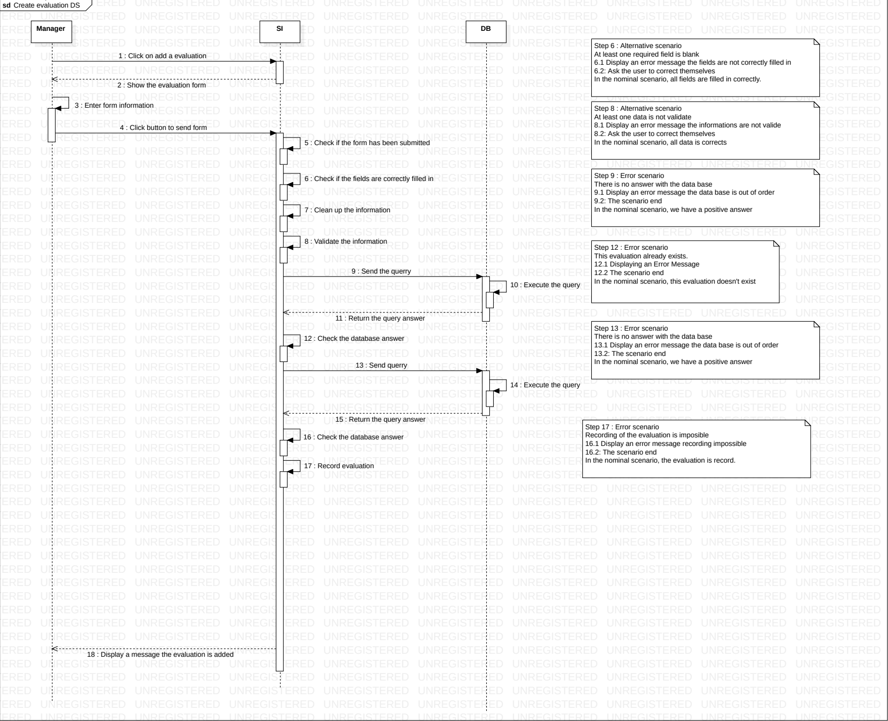
Diagramme de Séquence :Create evaluation DS::Interaction1::Create evaluation DS
