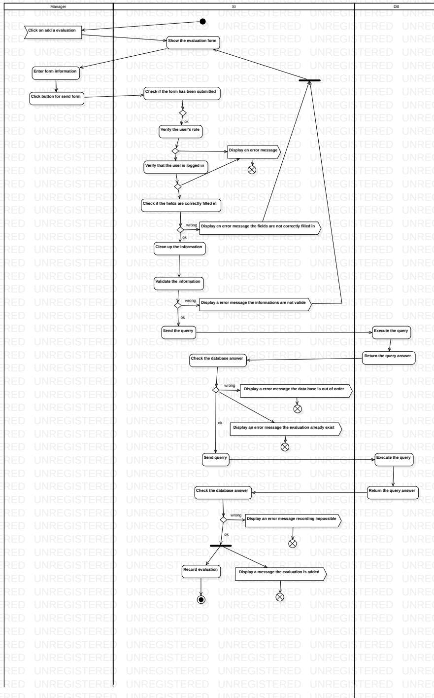
Diagramme d'Activité : Create evaluation DA: Create evaluation DA
