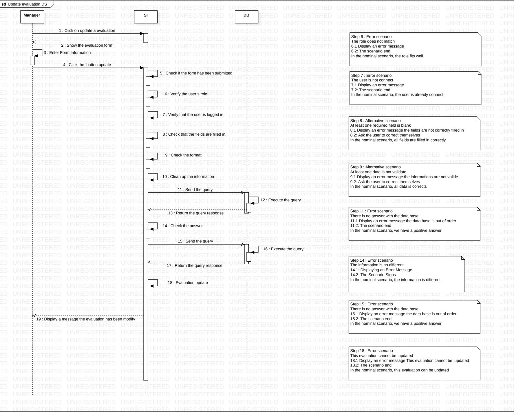
Diagramme de Séquence::Update evaluation DS::Interaction1::Update evaluation DS
